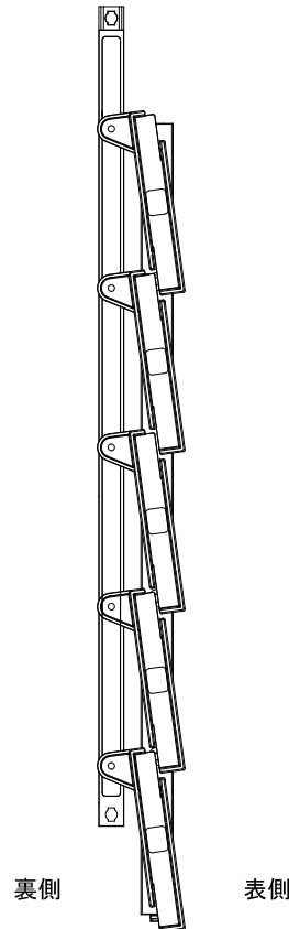
側面図 閉じた状態
